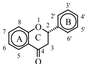
(7) Flavanone
