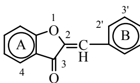
(5) Aurone
