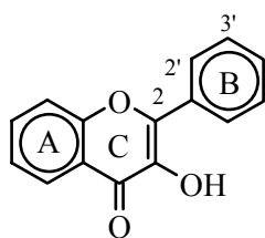
(9) Flavonol
