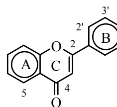
(8) Flavone
